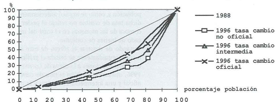
Gráfico 6 - Aproximaciones a la curva de Lorenz. Ciudad de La Habana.
