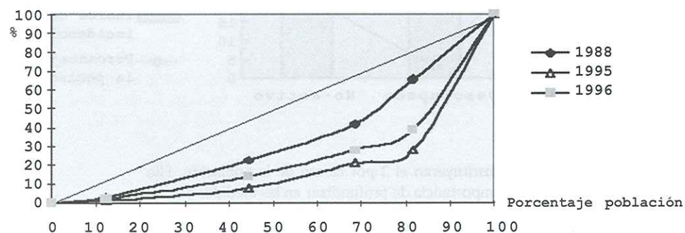
Gráfico 5 - Distribución de los ingresos. Aproximaciones a la curva de Lorenz. Ciudad de La Habana.
