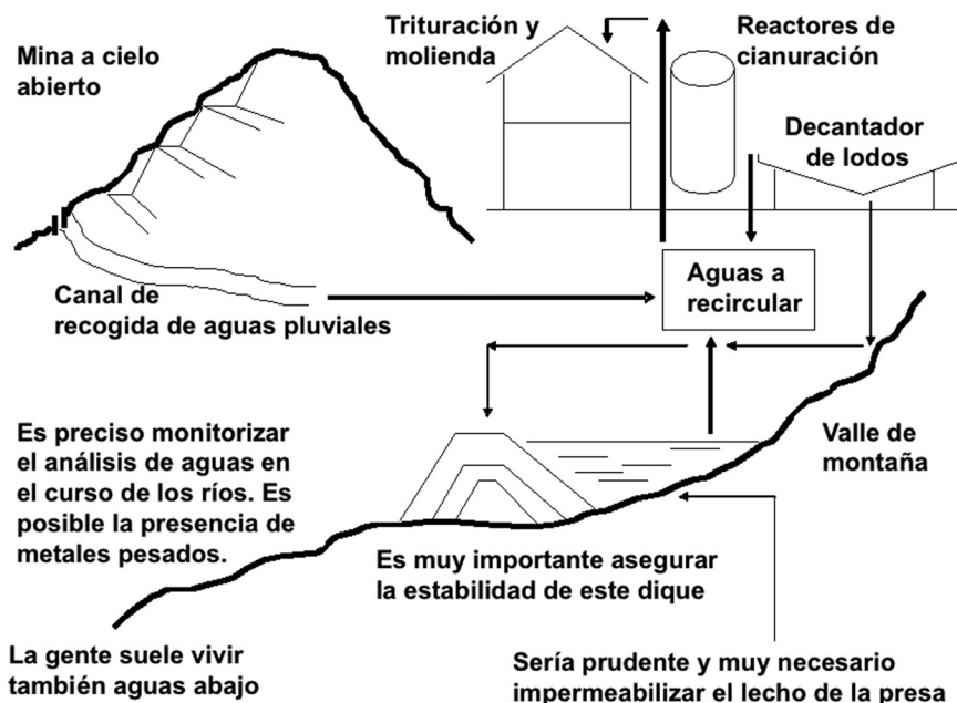
Figura nº 2.- Esquema de minería y extracción de oro
