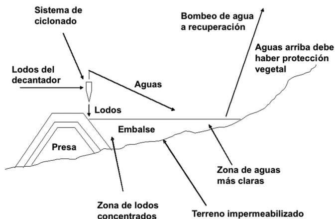
Figura nº 3.- Esquema de una presa de lodos prevista para recirculación de aguas
